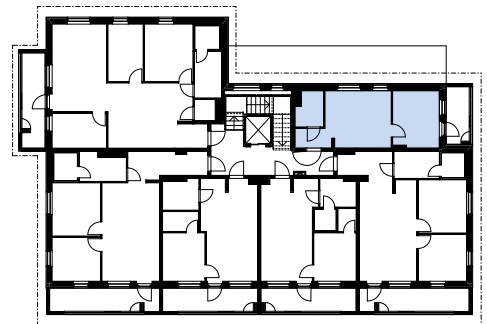
Pohjapiirustus 2.krs 1:500
