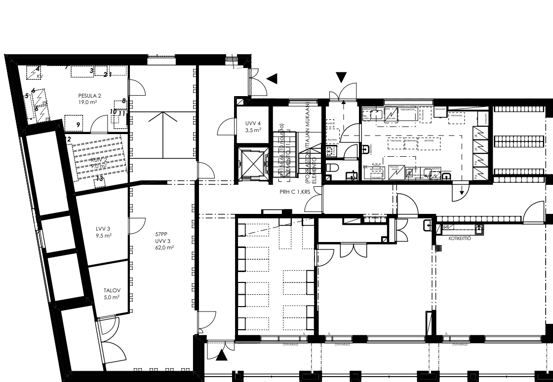
1:200 1. KERROS, PRH C
