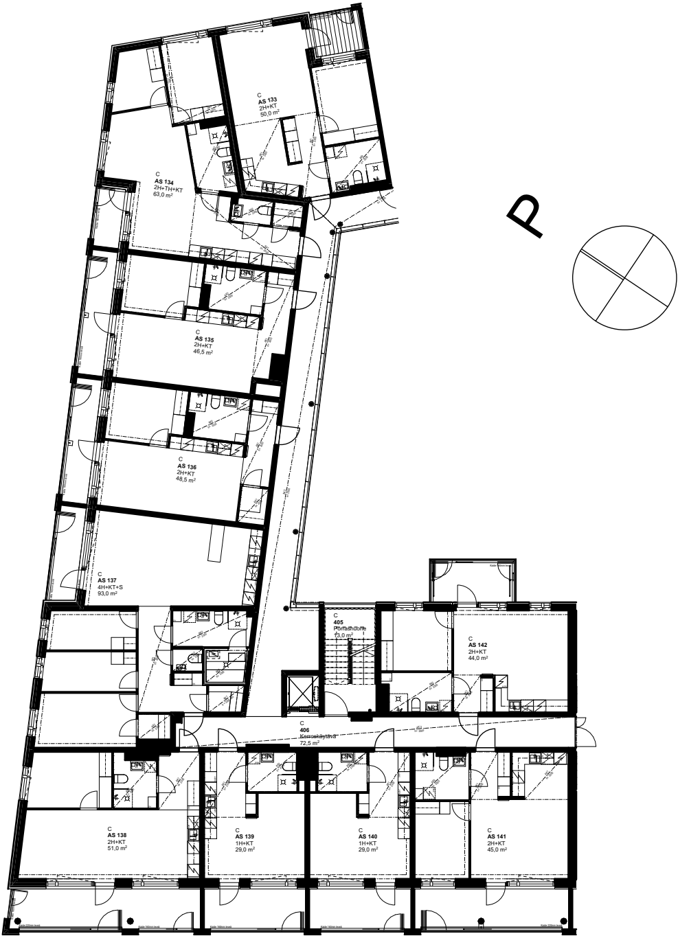
3.-4. krs
