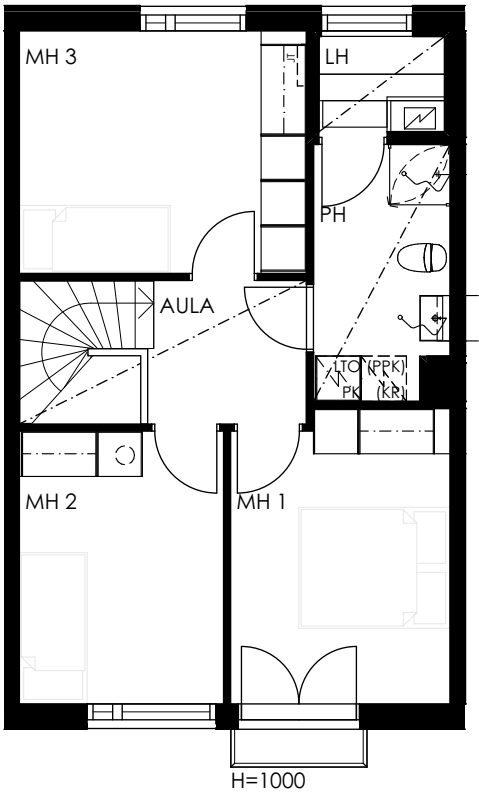
2. KERROS
