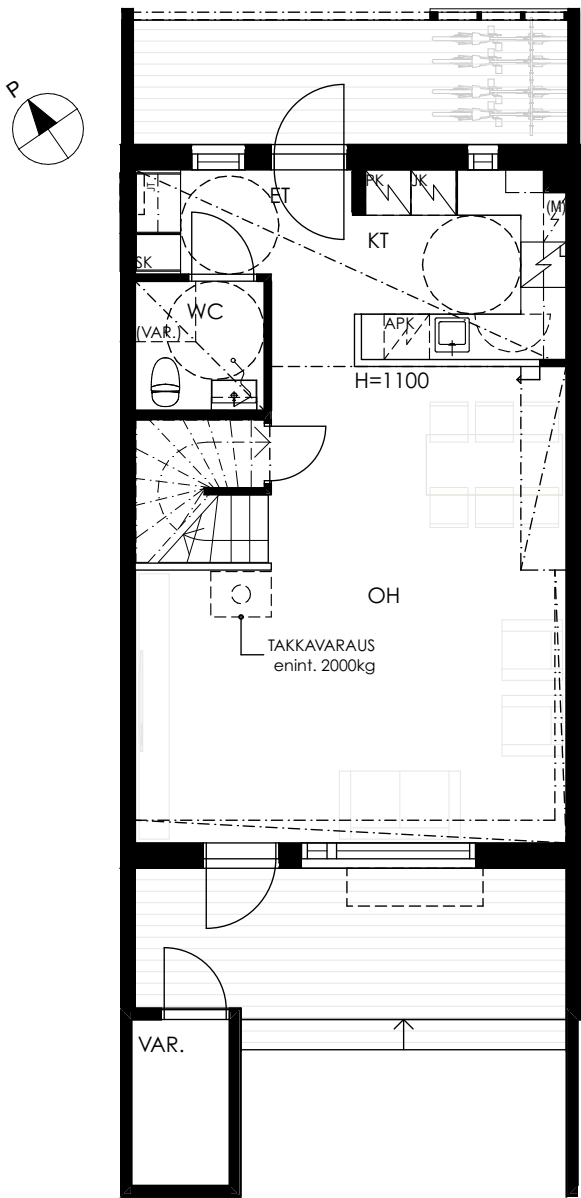
1. KERROS
