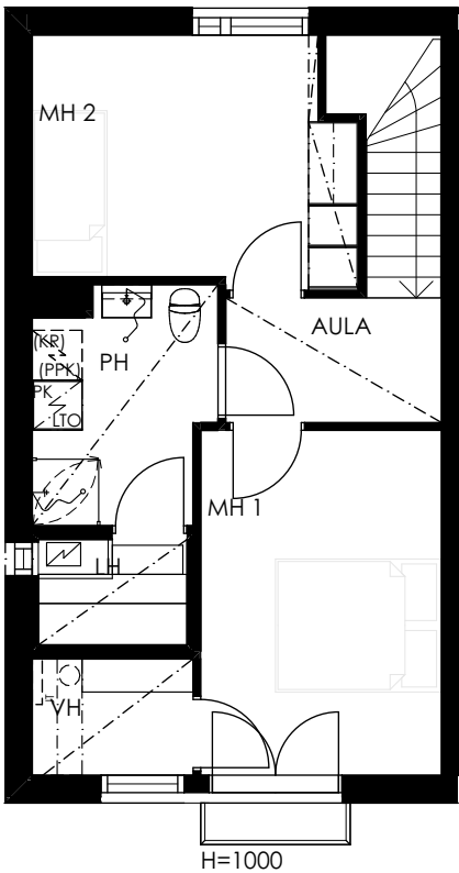
2. KERROS
