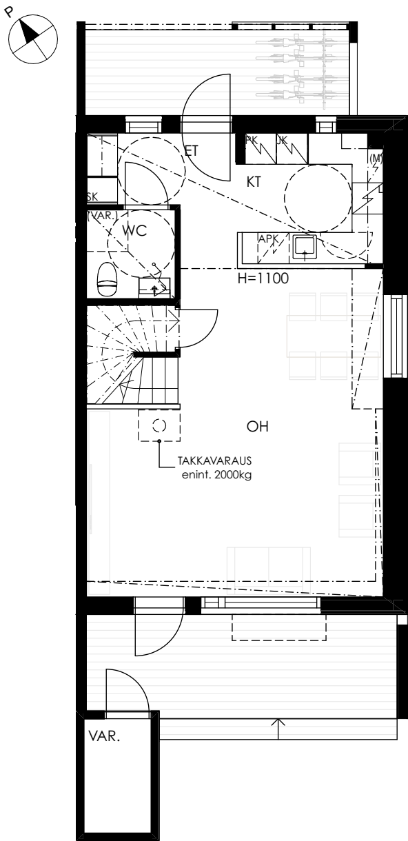
1. KERROS
