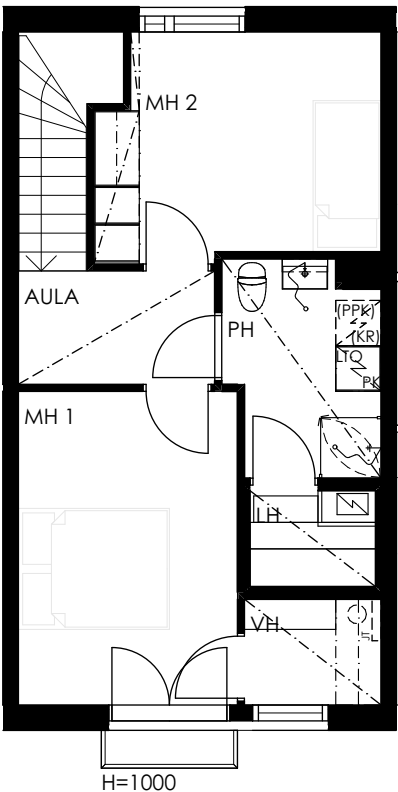
2. KERROS
