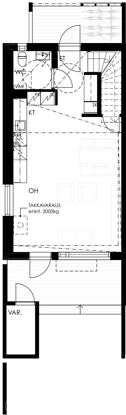
1. KERROS
